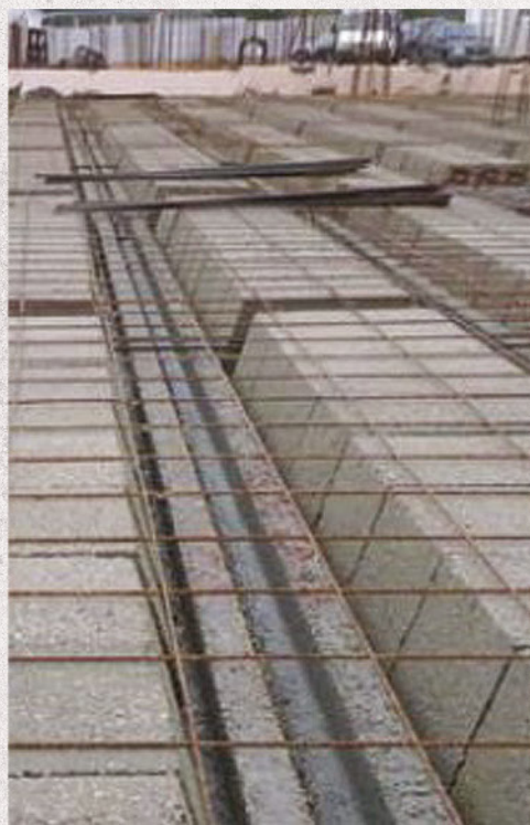
Travetti e Pignatte
